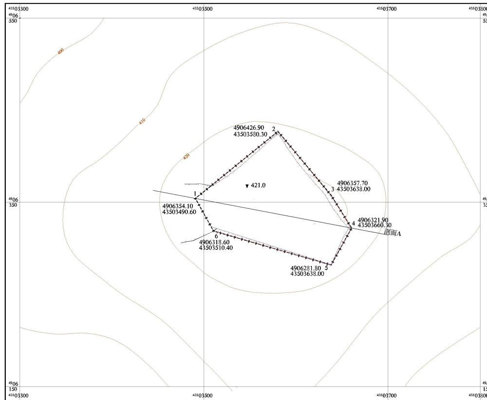
黑龙江省宁安市海浪镇八良子村庙岭山山砂场建筑用砂矿开采終了平面图
