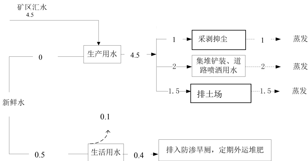
图3-2-1 水平衡图 单位 (t/d)
