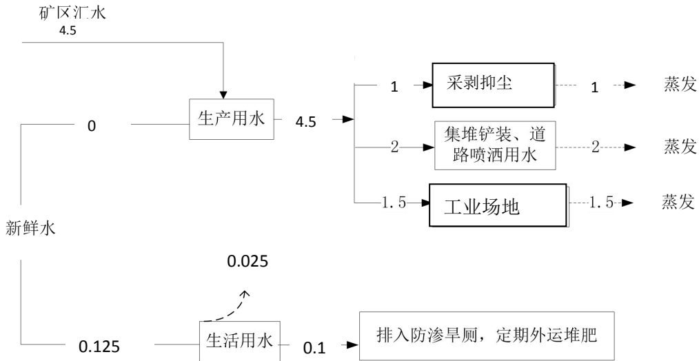
图3-2-1 水平衡图 单位 (t/d)
