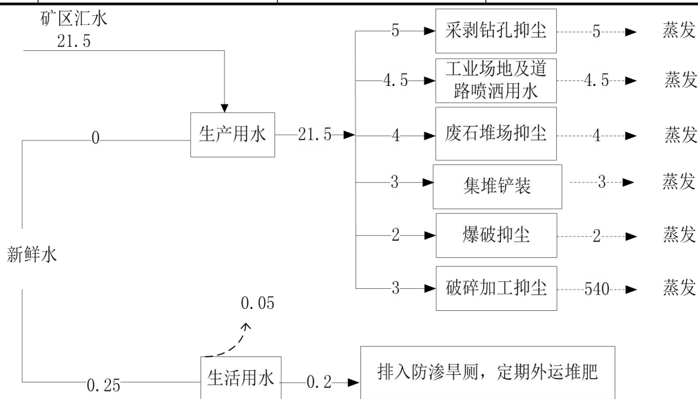
图3-2-1 水平衡图 单位 (t/d)
