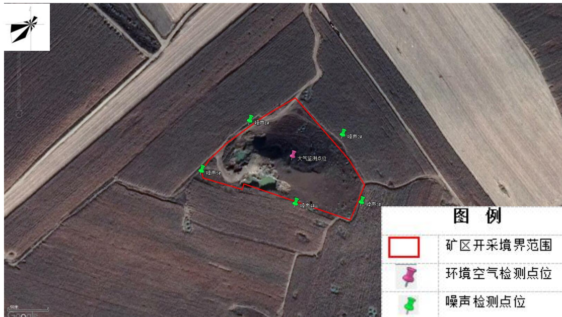
图4-3-1 监测点位布设图
