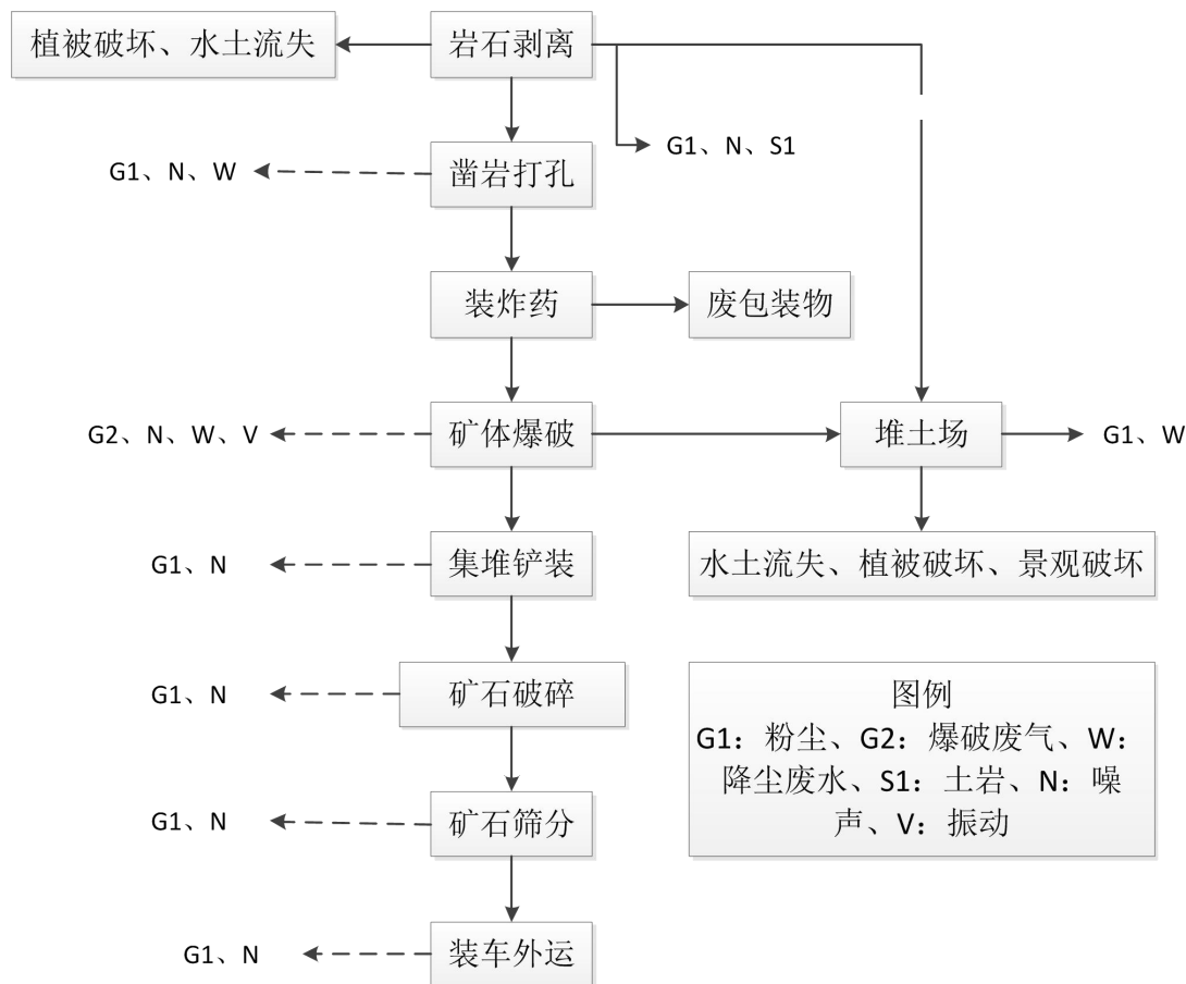
图3-3-1 本工程工艺流程及产污环节示意图
