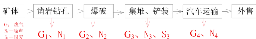
图 3-3-1 本项目工艺流程及产污环节示意图
