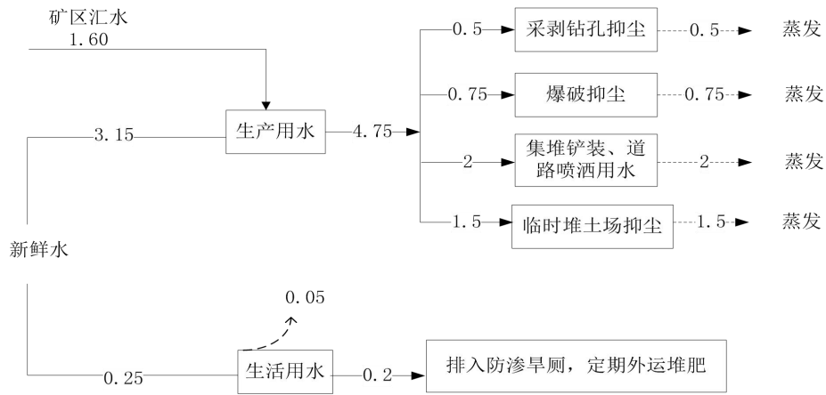
图 3-2-2 水平衡图 单位 (t/d)
